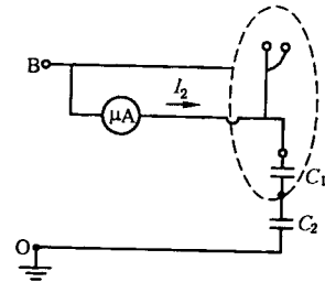
b) 流经人体电流测量原理图
